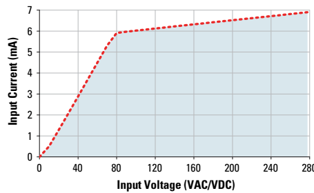
90-280 VAC/VDC Input
