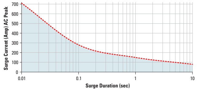
DR2260x30x
