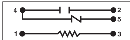
SPDT
