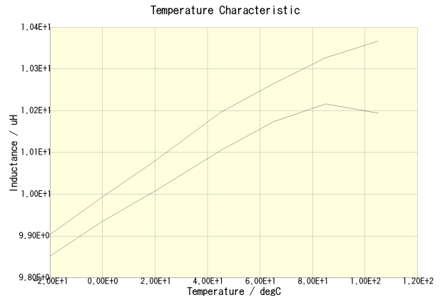
NLCV32T-100K-PF(DC = 0A)
