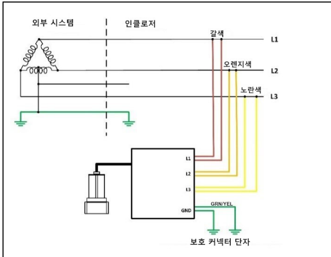
하이 레그 DELTA: 3와이어 + 중립 + PE
