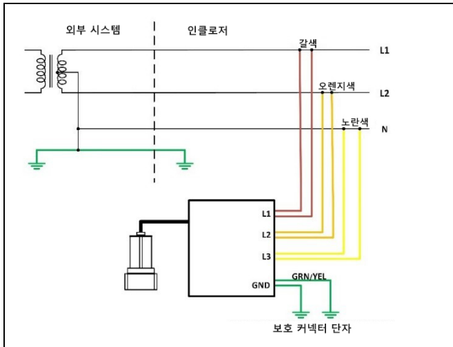
단상: 3와이어 + PE
