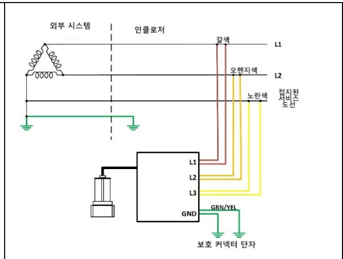
모서리 접지 DELTA: 3와이어 + PE
