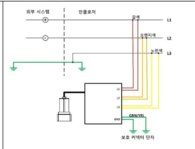
DC 시스템: 2와이어 + PE
