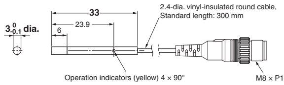
E2E-C06N04-CJ-□□
