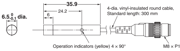
E2E-S05N03-CJ-□□
