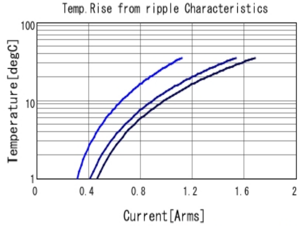
GRM188R71C104KA01 Temp. rise ■ 400kHz ■ 800kHz ■ 1MHz
