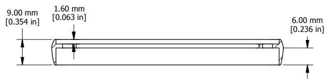
OPEN BEZEL
