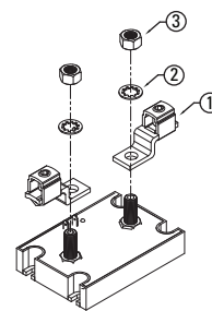
fig. 2 Lug Terminal Connections
