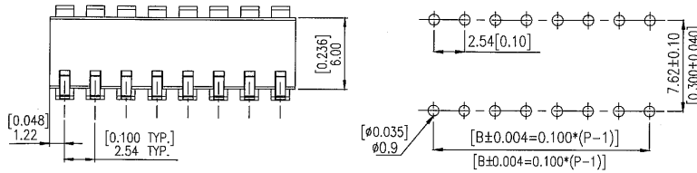
P.C.B. LAYOUT
